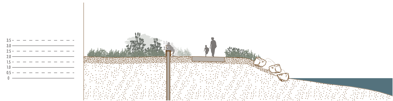
Tværsnit mod syd, med synlig klimasikring, som træbeklædt spuns langs promenade
