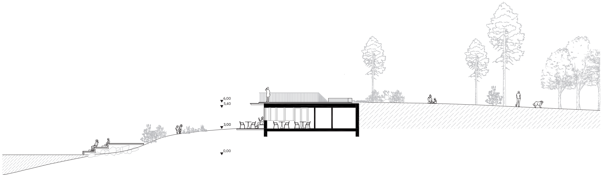
Strandbar, snit DD 1:250
