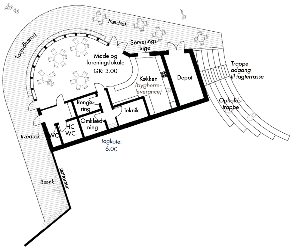
Stueplan 1:250 som viser strandbarens faciliteter
