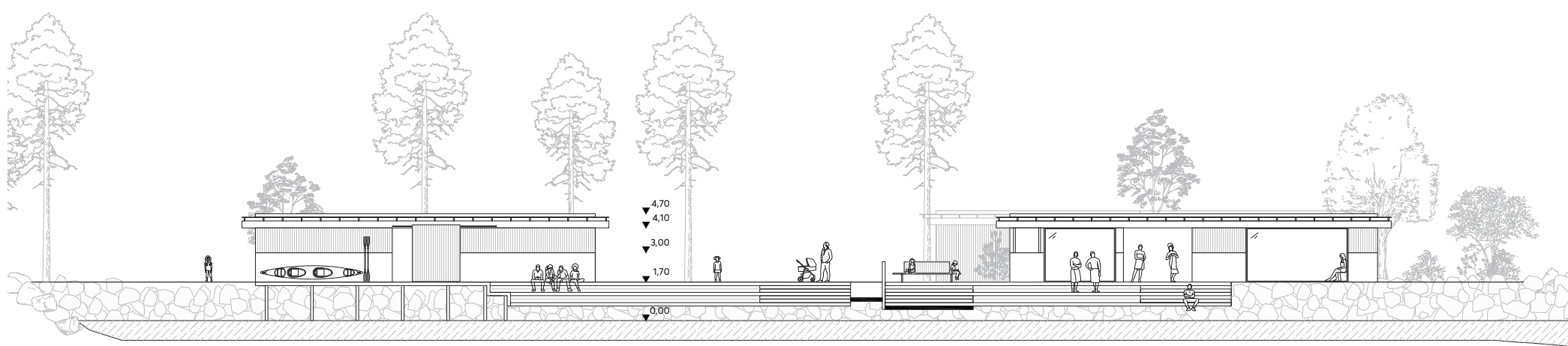
Opstalt BB set fra nord ind mod havnebadets trappeanlæg. 1:250
