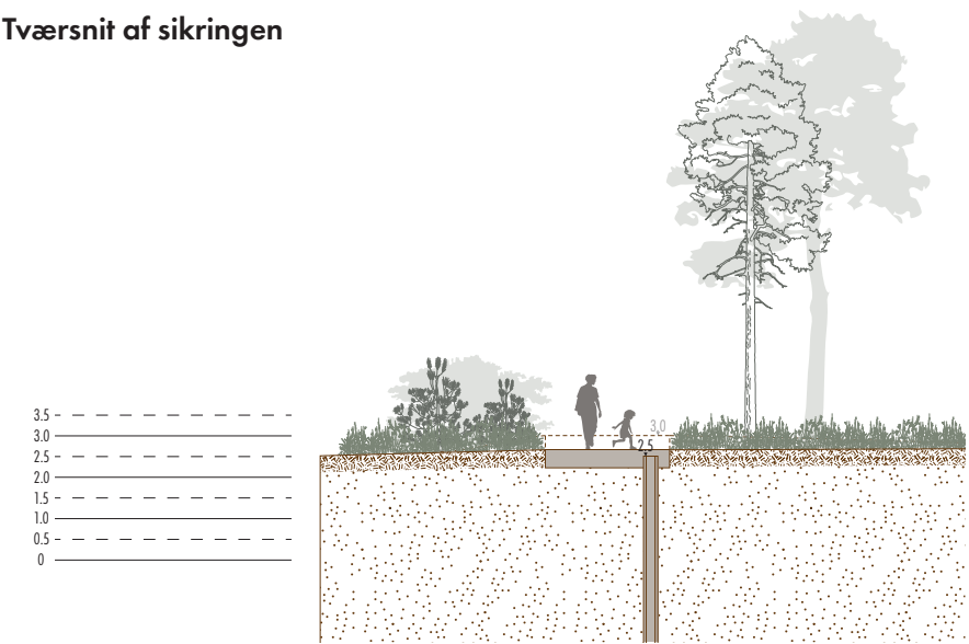
Tværsnit i park, med klimasikring under promenade
